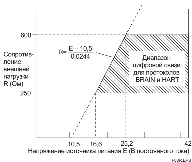
Рис. 2 Взаимосвязь между напряжением источника питания и сопротивлением внешней нагрузки (Выходной сигнал с кодами D и J)
